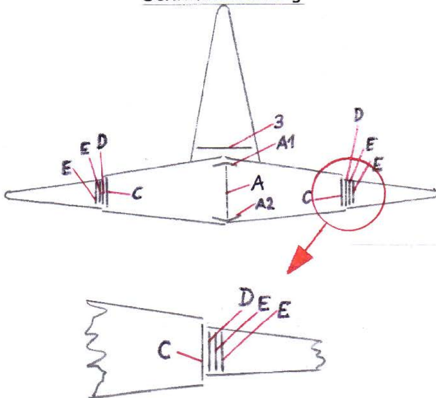
Schnittzeichnung
