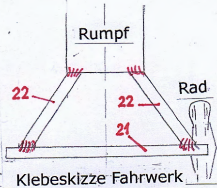
Verspannung grün
