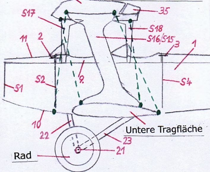
Verspannung grün
