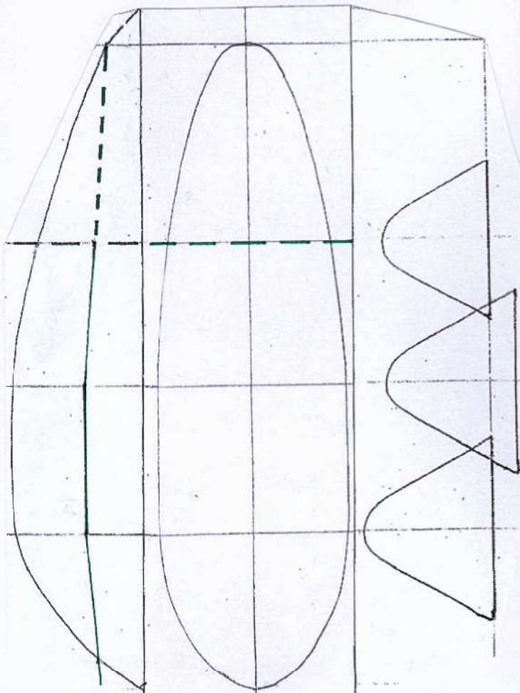
Schema für Tiefziehform
