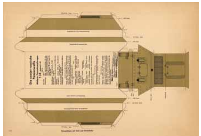
Modell Nr. 1: Die sowjet-russische Panzerwaffe, Mittlerer Panzerkampfwagen T 34, Maßstab 1:20, 4 Bogen 35 x 50 cm, Datum 15.2.42.
